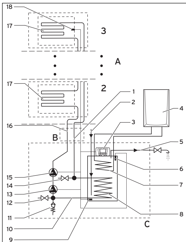
Abb. 2.3 Composants principaux du système HelioSet avec ballon S-FE 350 SC P (schéma de principe sans accessoires de raccordement)
