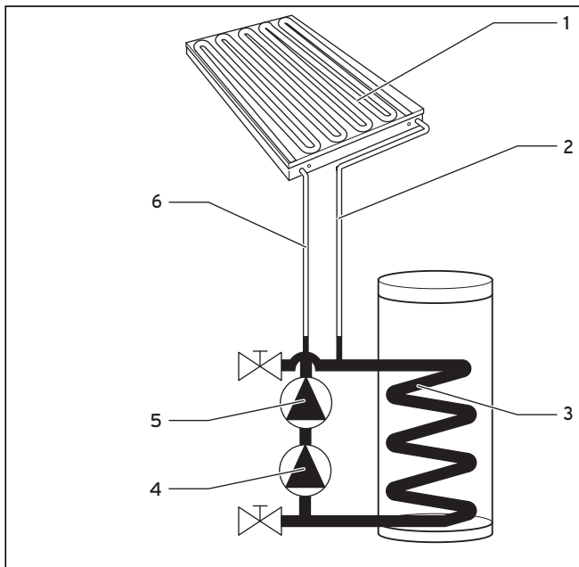
Abb. 2.1 Répartition du fluide caloporteur en cas d'arrêt de la/des pompe(s) du capteur
