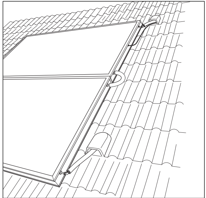
Abb. 2.4 2ème champ de capteurs HelioPlan SRD 2.3 en montage sur toiture
