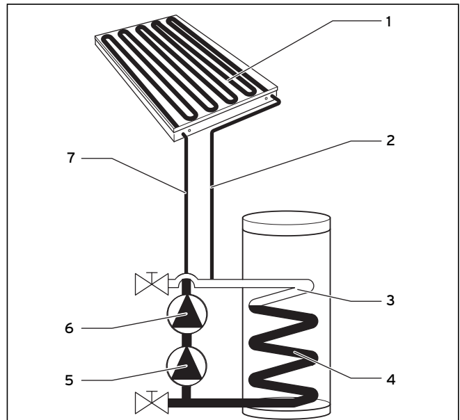
Abb. 2.2 Répartition du fluide caloporteur en cas de fonctionnement de la/des pompe(s) du capteur
