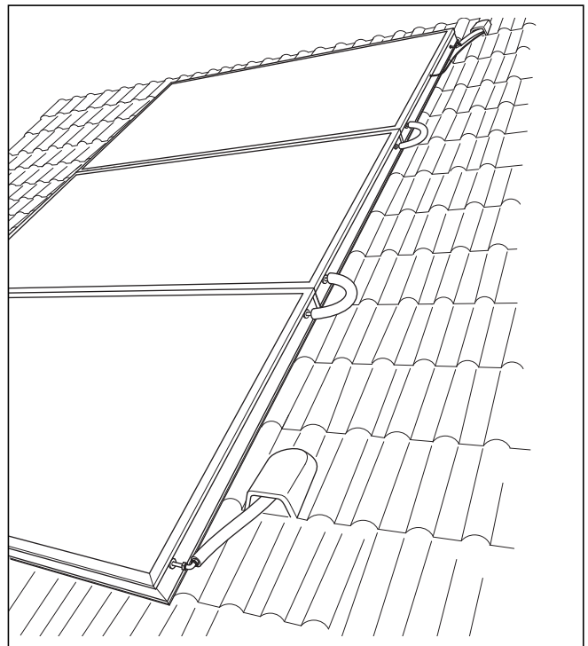
Abb. 2.5 Ternaire champ de capteurs HelioPlan SRD 2.3 en montage sur toiture
