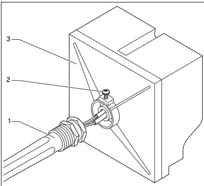
1 Tube de la sonde 2 Vis 3 Thermostat
