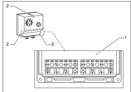
1 Bornes de raccordement 2 Vis
