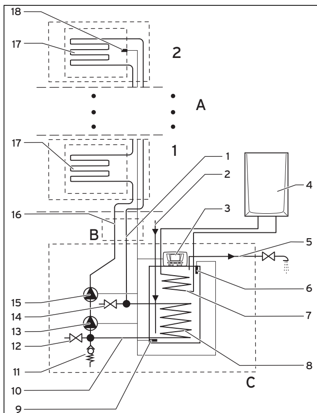
Abb. 2.3 Composants principaux du système HelioSet avec ballon S-FE 250 SC P oder 350 SC P (schéma de principe sans accessoires de raccordement)
