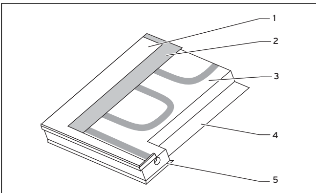
Abb. 2.7 Coupe du capteur plan Saunier Duval HelioPlan SRD 2.3
