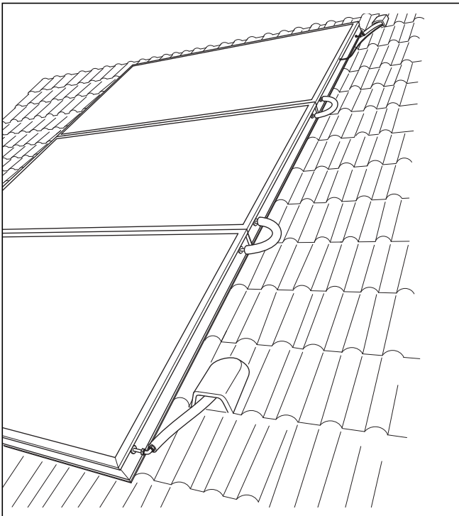
Abb. 2.6 Ternaire champ de capteurs HelioPlan SRD 2.3 en montage sur toiture
