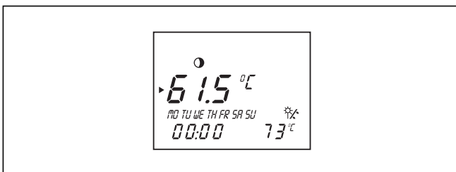
Abb. 4.5 Choix de la température de consigne du ballon solaire
