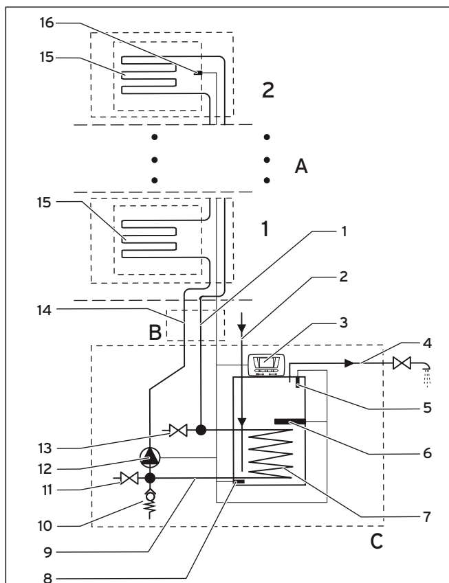
Fig. 2.3 Principaux composants du système HelioSet avec ballon S-FE 250 SE (schéma de principe sans accessoires de raccordement)
