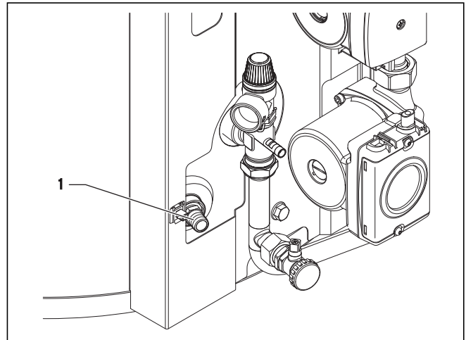
Abb. 4.2 Soupape de vidange pour ballon d'eau potable
